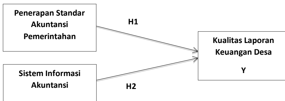
Gambar 2.1 Rerangka berpikir
