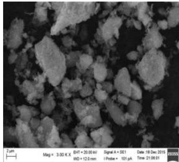
Gambar 3 Morfologi permukaan zeolit alam
