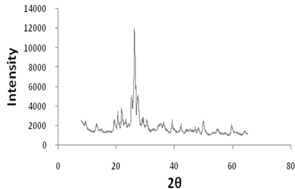
Gambar 1 Difraktogram Zeolit Alam Ende
